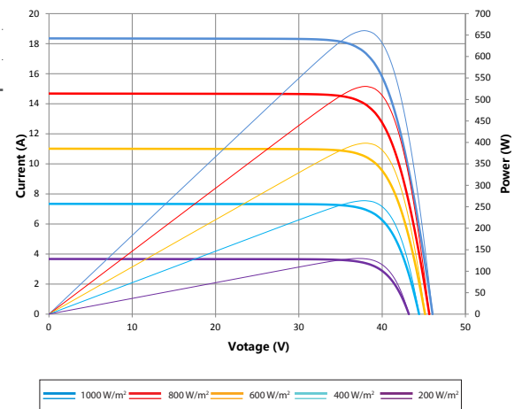
电流-电压 & 功率-电压曲线图 (660S)
